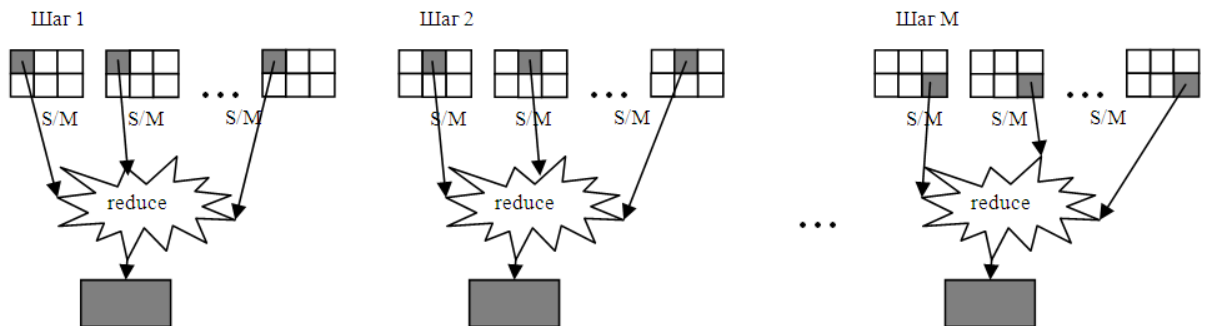
Рис. 2. Схема компоновки изображения для мультidisплейного комплекса с использованием MPI-операции reduce
