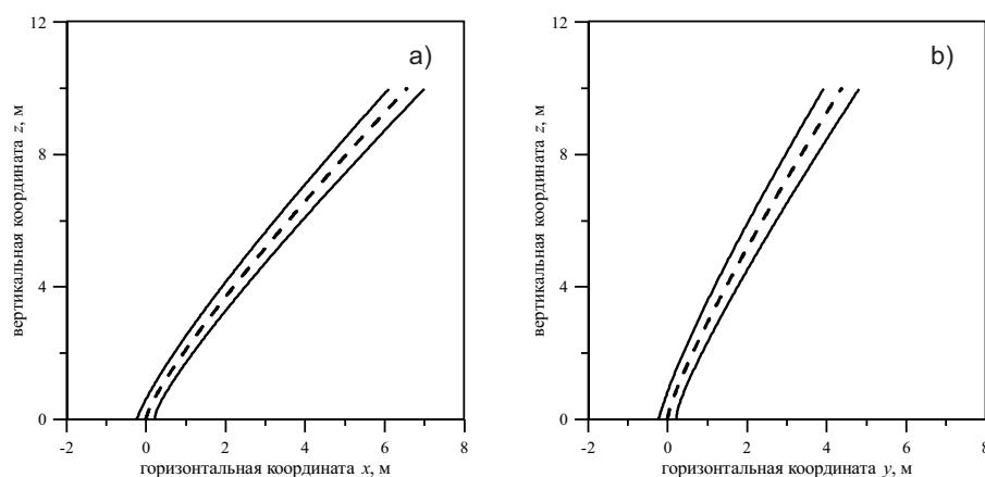
Рис. 2. Траектория струи
