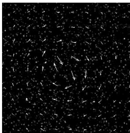
Рис. 3. Поле скорости потока в жидкости, определенное с помощью стандартного кросскорреляционного алгоритма
