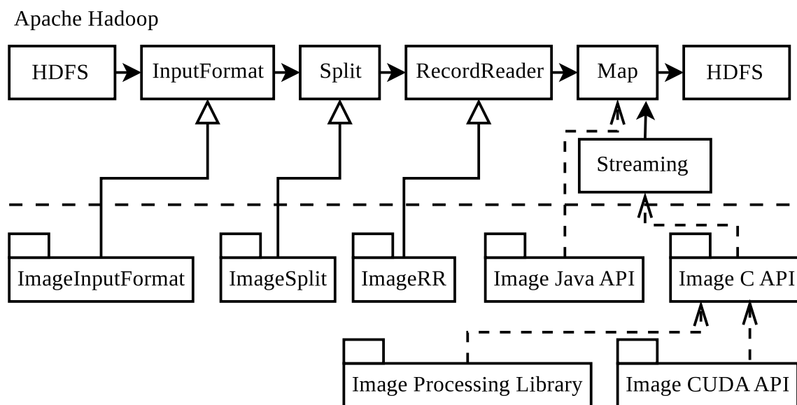
Рис. 1. Логическая архитектура системы обработки изображений с автоматическим распараллеливанием на основе Hadoop
